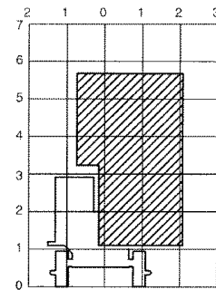
11) HORIZONTAL DRILLING
